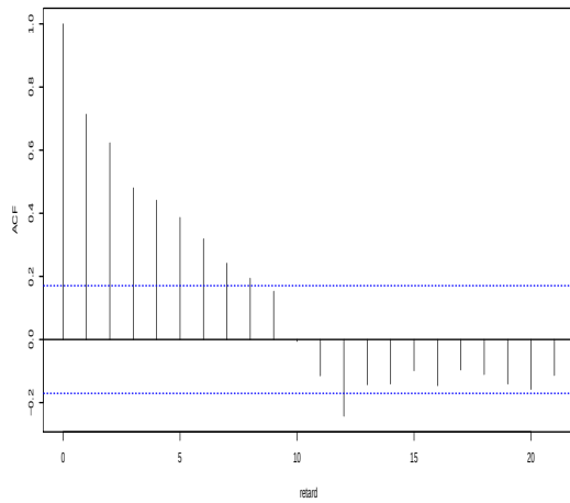
FIGURE 3.12 – ACF de la série différenciée et sortie R pour le test de Dickey-Fuller
