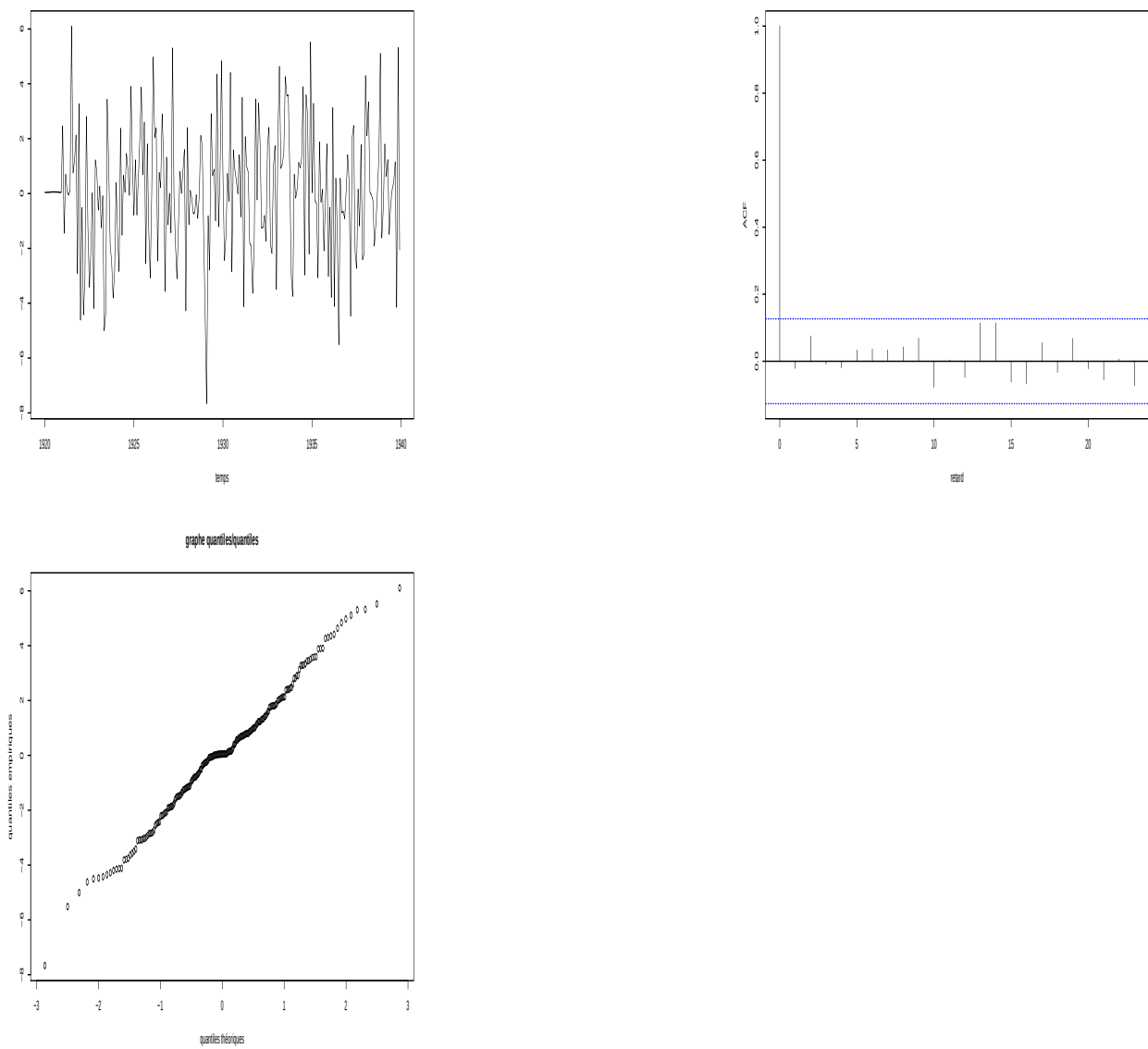
FIGURE 3.6 – graphe des résidus, ACF des résidus et comparaison des quantiles des résidus avec ceux d’une gaussienne
