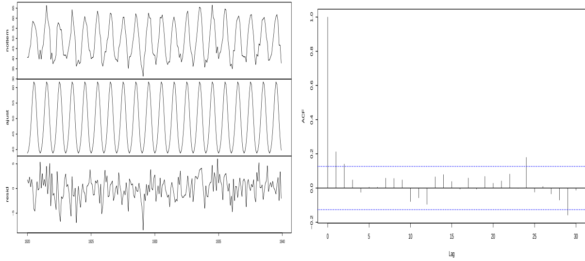
FIGURE 2.1 – Série temporelle désaisonnalisée par régression et autocorrélation des résidus obtenus (sur la figure de droite la barre n° i représente la valeur du coefficient de corrélation empirique entre (x_1, \dots, x_{T-i}) et (x_{i+1}, \dots, x_T) ).
