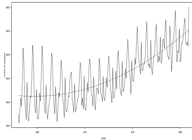
FIGURE 1.7 – Tendance estimée pour la deuxième régression (en pointillé)
