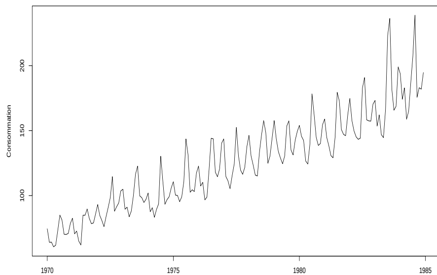
FIGURE 1.2 – Consommation mensuelle d'électricité (en kwh) entre 1970 et 1985
