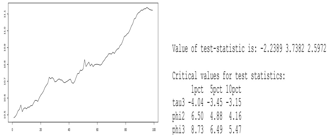
FIGURE 3.10 – Logarithme de la dépense de consommation trimestrielle au Royaume-Uni et sortie R pour le test de Dickey-Fuller
