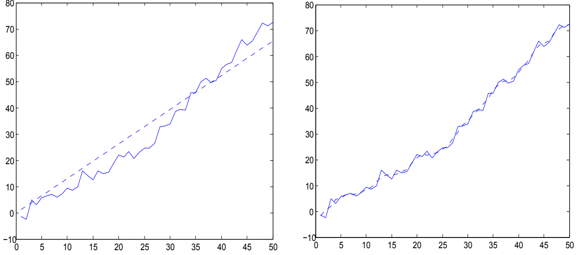
FIGURE 1.8 – Estimation de la tendance par régression (en ignorant la rupture, graphe de gauche) puis par l'application de M(X)_t = \frac{X_{t-1} + X_t + X_{t+1}}{3} qui conserve les droites (la tendance estimée figure en pointillés)
